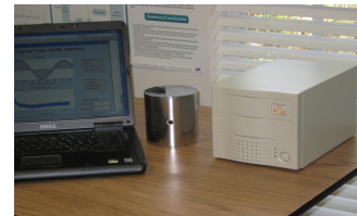
iSpin-NMR
